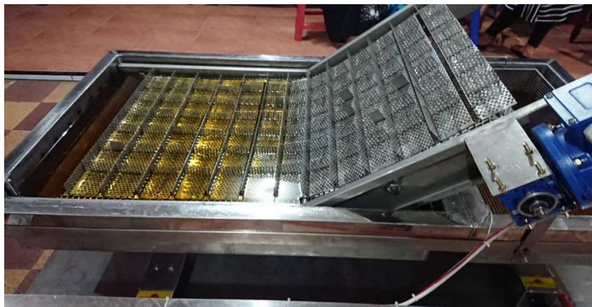
Gambar 3. 24 Mesin Penggoreng Tempe
